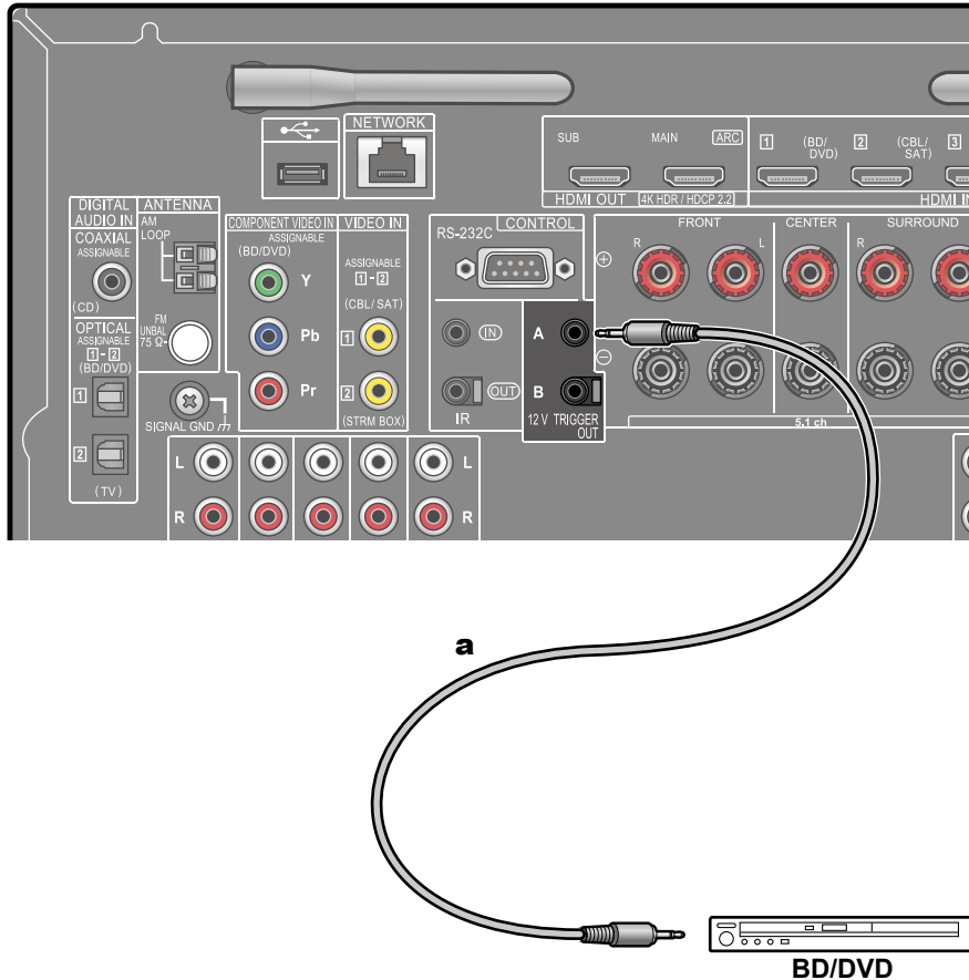
a Monaural mini plug cable ( \phi 1/8"/3.5 mm)
