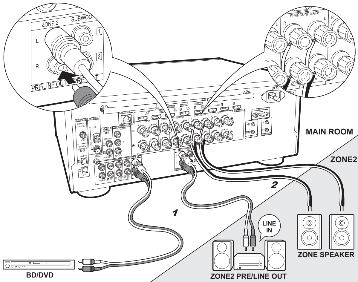
1 Cable de audio analógico, 2 Cable de altavoz
