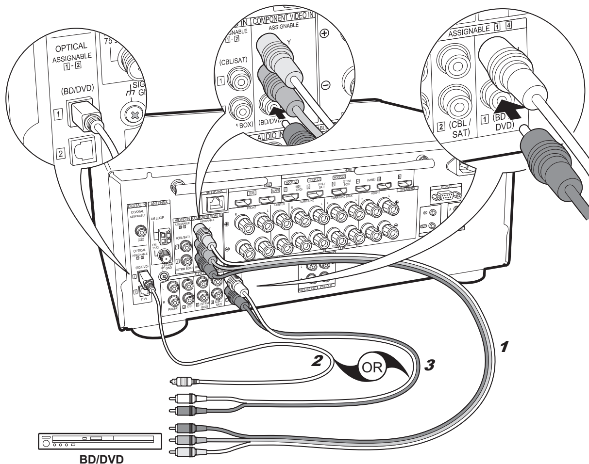
1 Cable de video componente, 2 Cable óptico digital, 3 Cable de audio analógico
