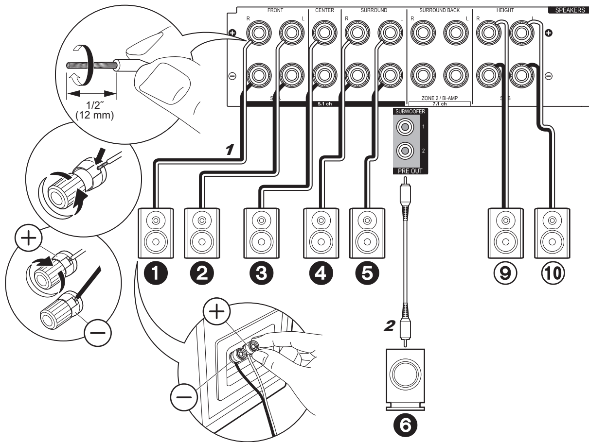
1 Cable de altavoz, 2 Cable de subwoofer
