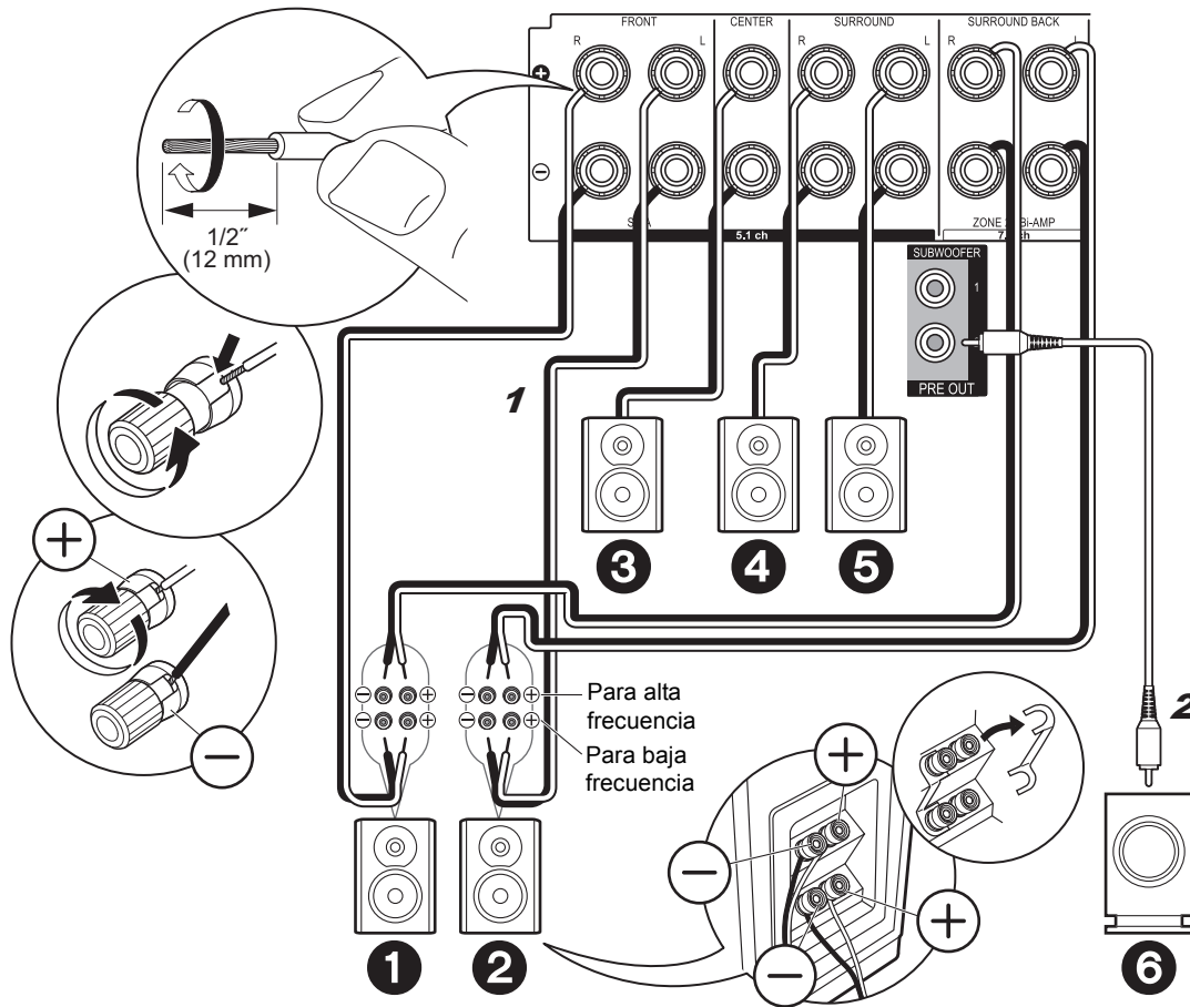
1 Cable de altavoz, 2 Cable de subwoofer
